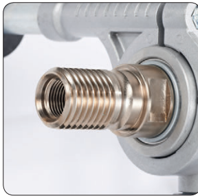
Combi-as, 1/2" G en 5/4" UNC
