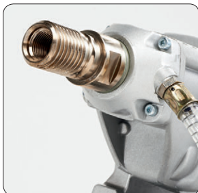
Combi-as, 1/2"G en 5/4"UNC
